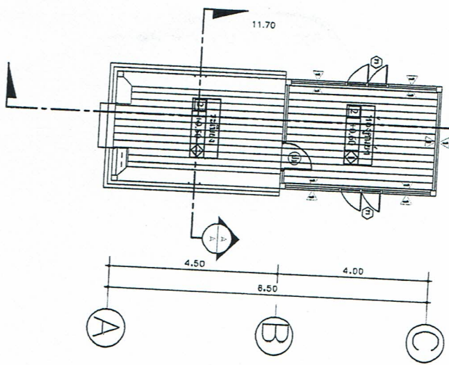
แปลนพื้น SCALE 1 : 100
